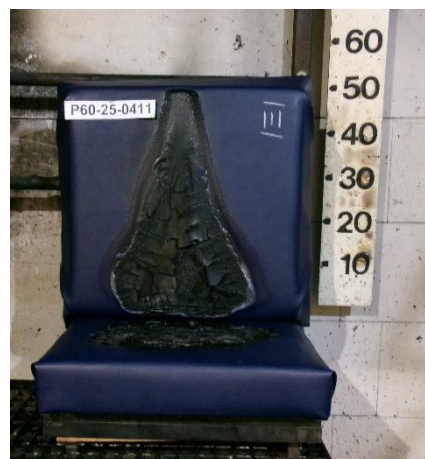
Abb.6: Sitz 3 nach der Prüfung Fig.6: Seat 3 after testing
